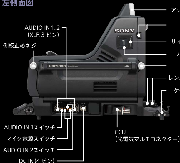
左側面図
