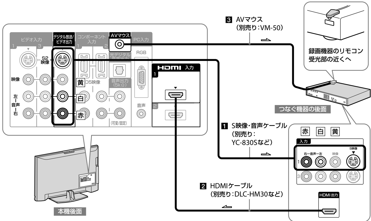
⇒:映像・音声信号の流れ
