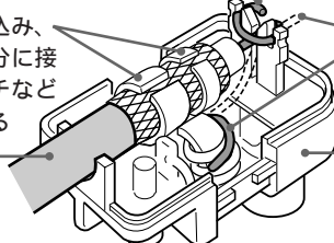
VHF/UHF用アンテナ コネクター
