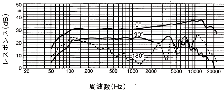
標準周波数特性
