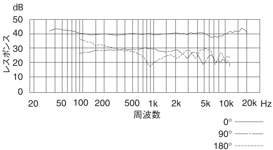
標準周波数特性
