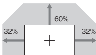
レンズシフト量 (VPL-FH35/FH30)
