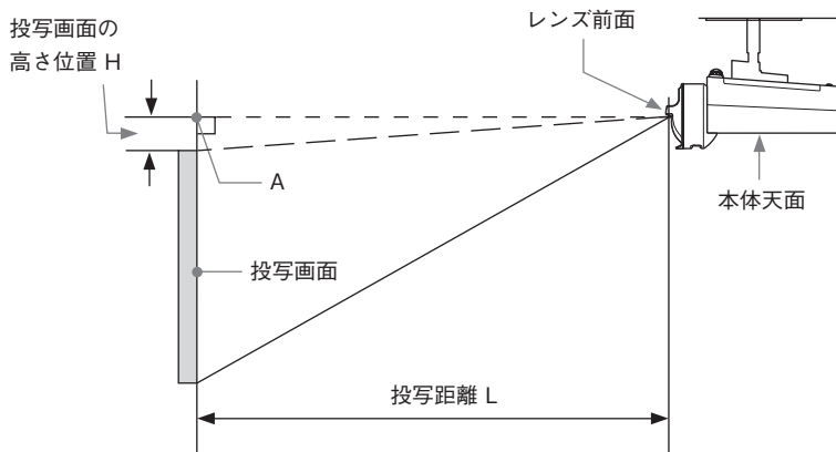
投写距離表 (アスペクト比 16:10)
