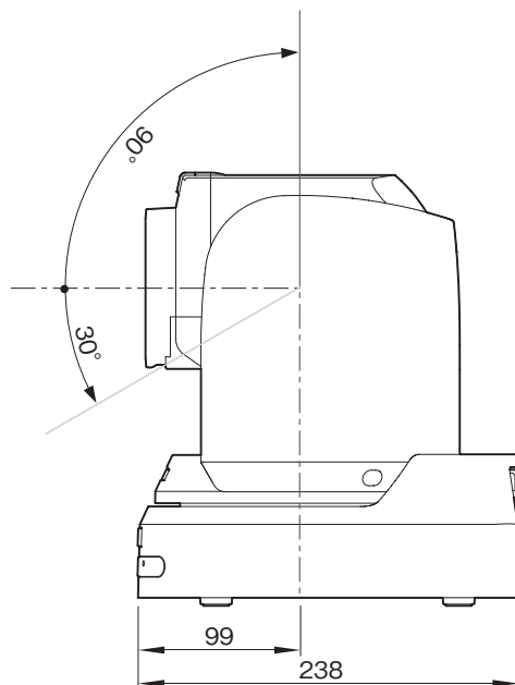
側面
