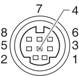
ピン配置図
