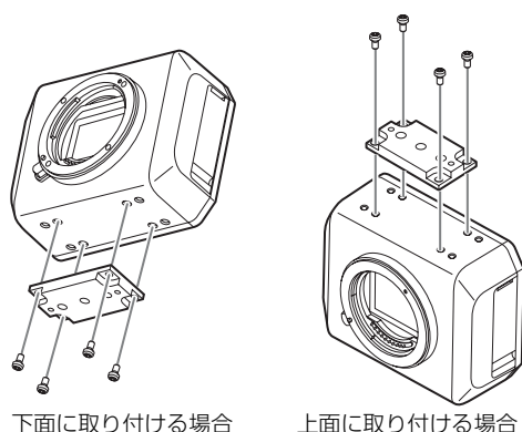
下面に取り付ける場合
