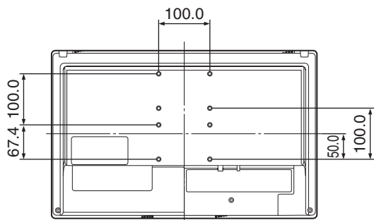
後面（モニタースタンド未装着時）
