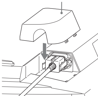
AC インレットカバー (付属品)
