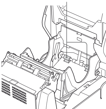
Rullo di alimentazione della carta
