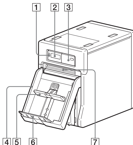
前面
