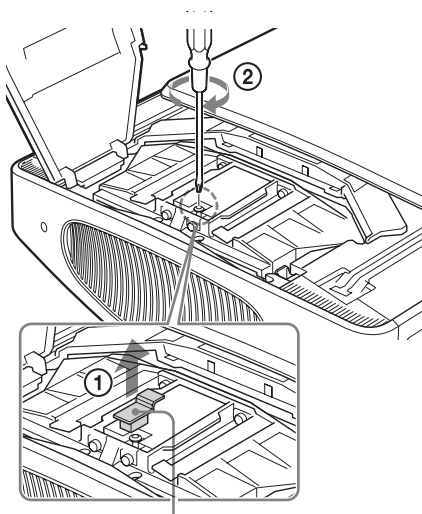
Capuchon de vanne
