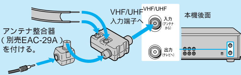
アンテナ混合器 (別売EAC-68) を付ける。
