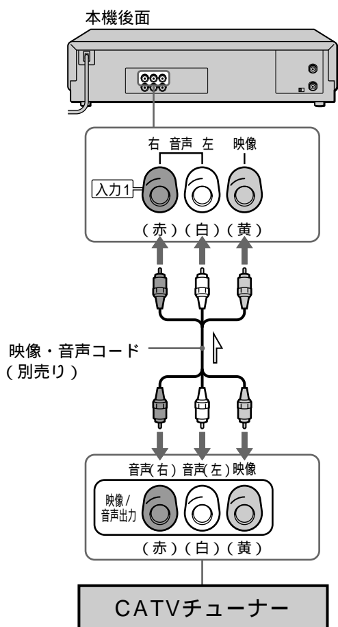
⇒ : 映像・音声信号の流れ
