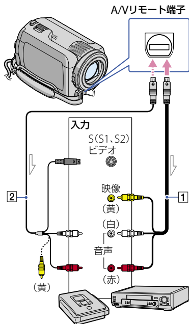
信号の流れ
