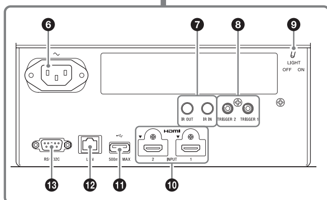
接続端子
