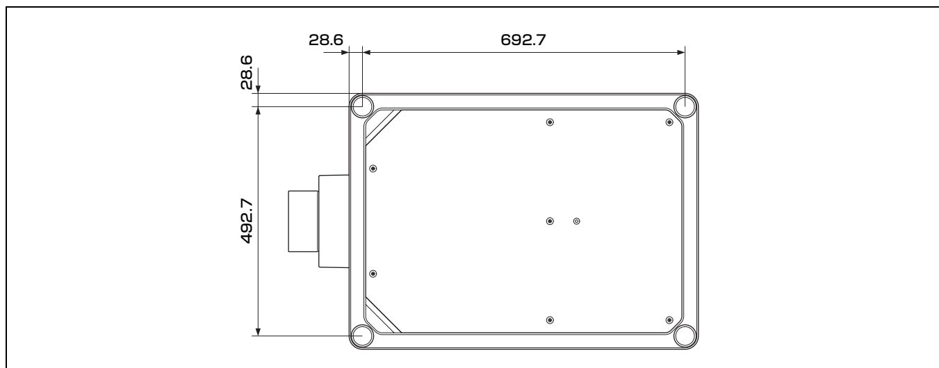
本体底面
