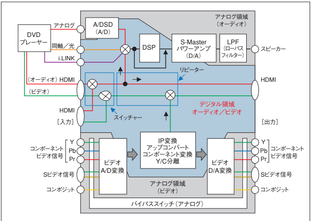
●図20: TA-DA9100ESの映像・音声の信号経路
