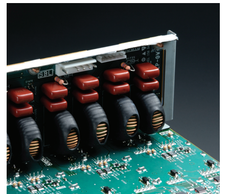
●写真8: ローパスフィルター部
