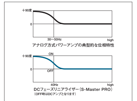
●図17: アナログアンプの位相特性をDSP演算によって再現
