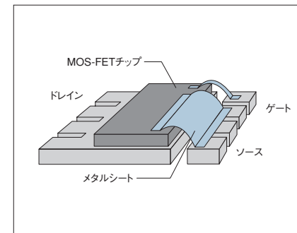
●図23: 大容量タイプのMOS-FETを採用した大電流
