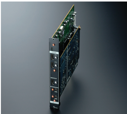
●写真5: 独立構成のHDMI基板(左)とi.LINK基板(右)
