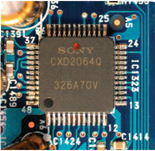
●写真4: A/VシンクIC、CXD2064
