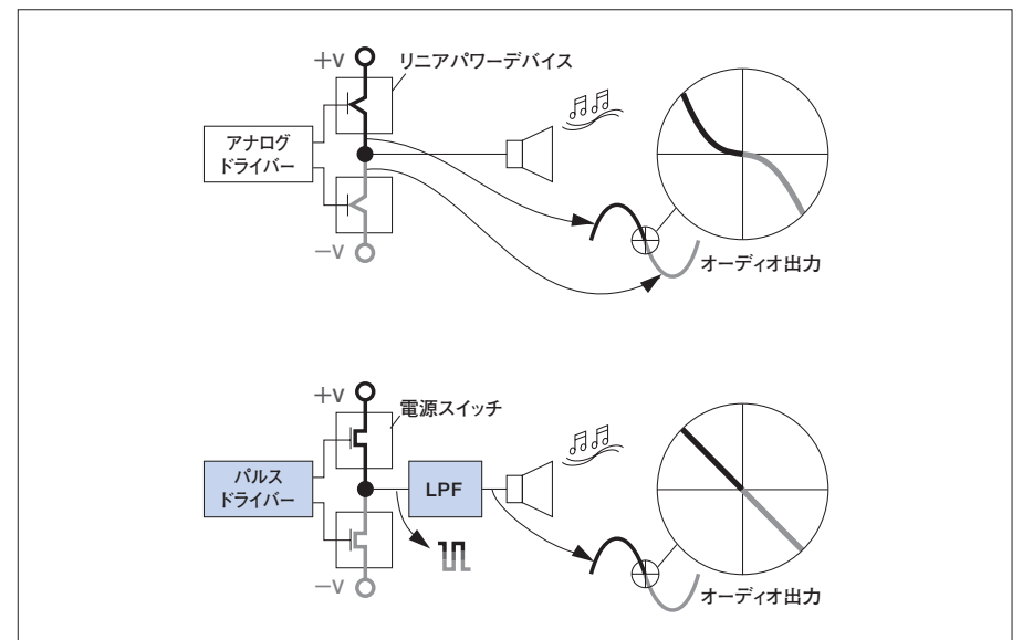
●図11: アナログアンプとS-Masterの出力波形の違い
