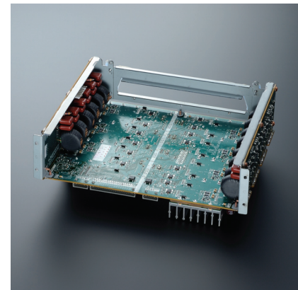
●写真7: パワーアンプブロックの裏側
