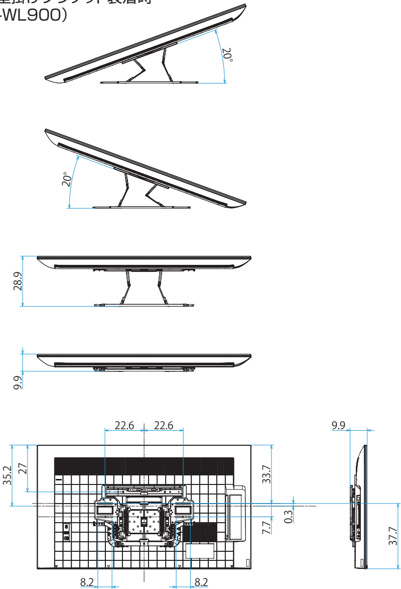
スリム壁掛けブラケット装着時 (SU-WL900)
