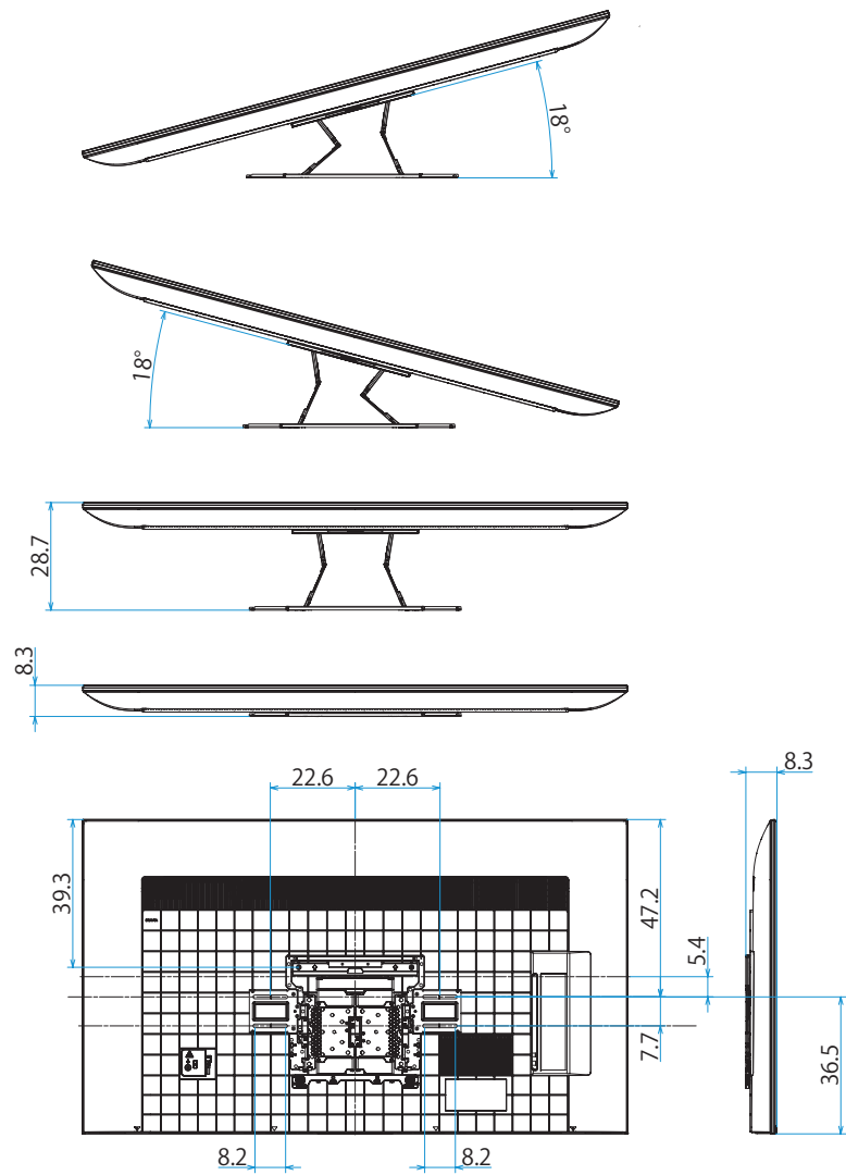
壁掛けブラケット装着時 (SU-WL850)
