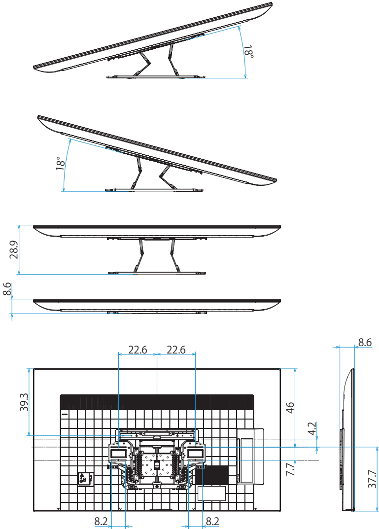
スリム壁掛けブラケット装着時 (SU-WL900)
