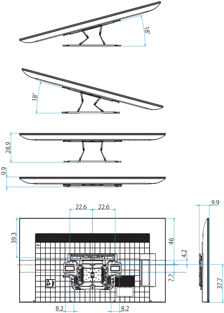
標準壁掛けブラケット装着時 (SU-WL900)
