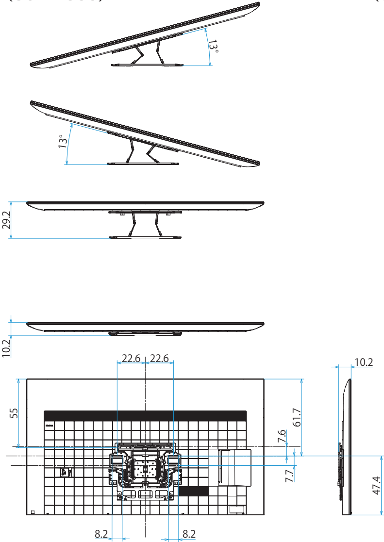
標準壁掛けブラケット装着時 (SU-WL900)
