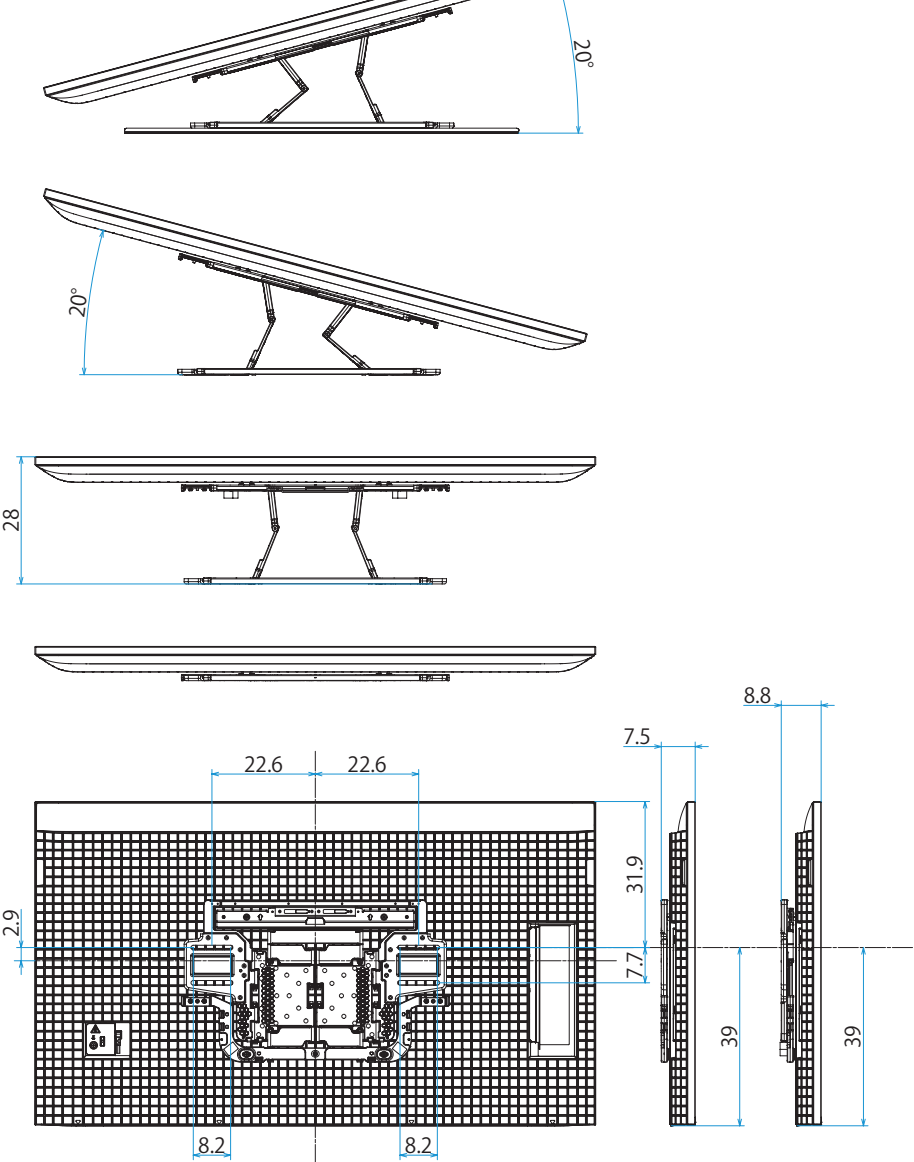
壁掛けブラケット装着時 (SU-WL900)
