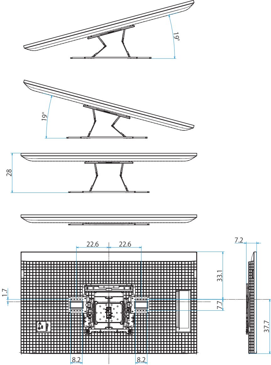
壁掛けブラケット装着時 (SU-WL850)
