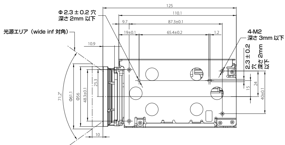
右側面
