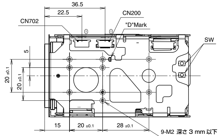
上面
