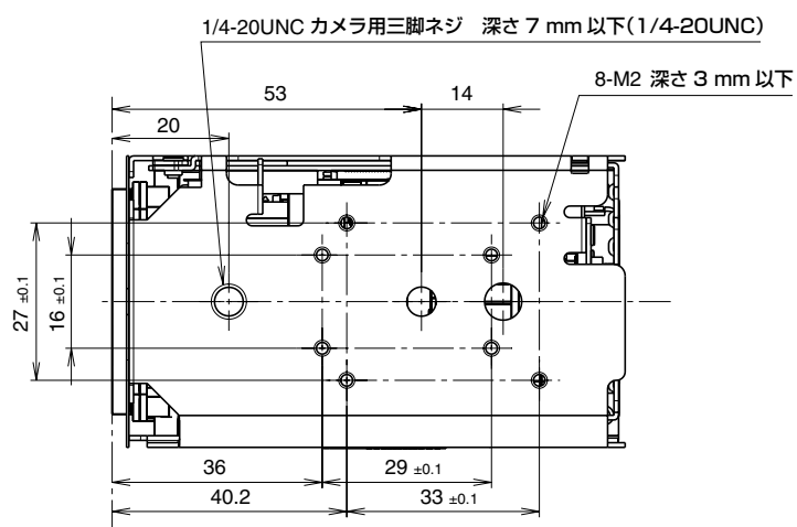
底面
