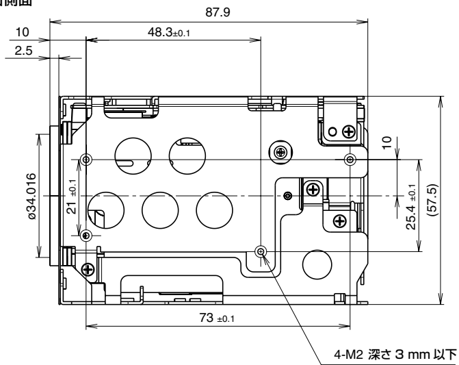
右側面
