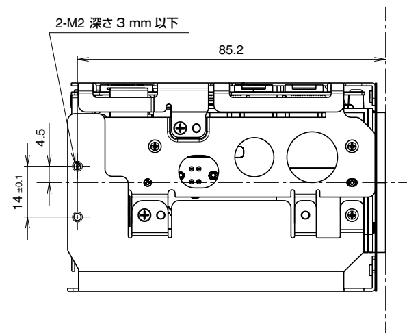
左側面
