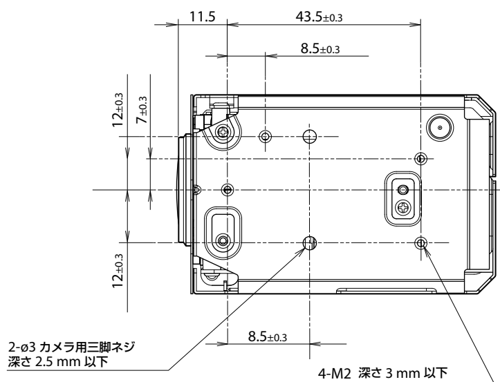
底面
