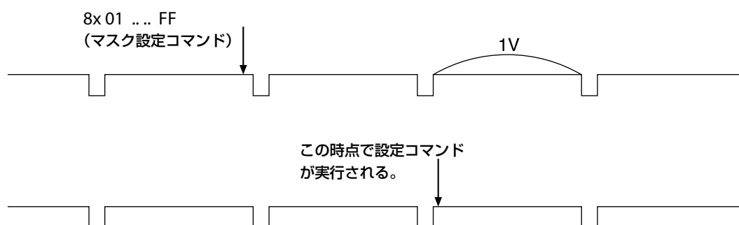
タイミングチャート
