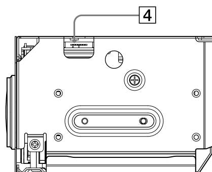
左側面
