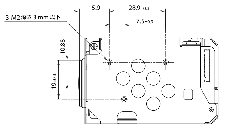
左側面
