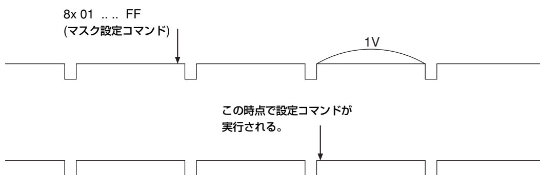
タイミングチャート
