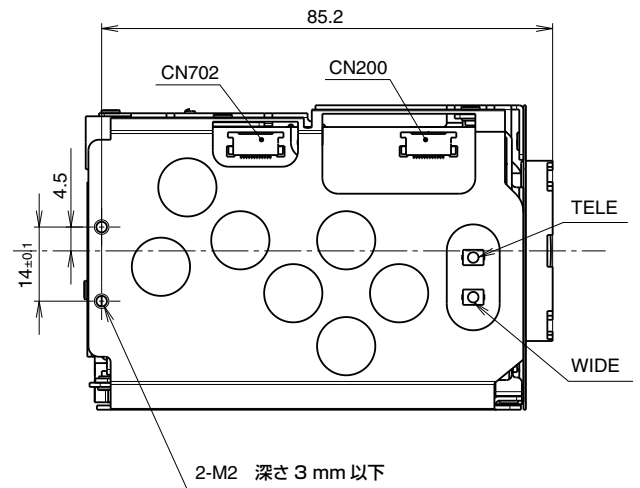
左側面
