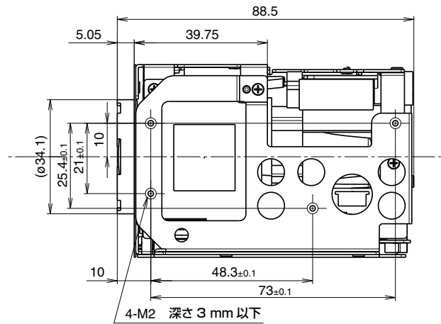
右側面
