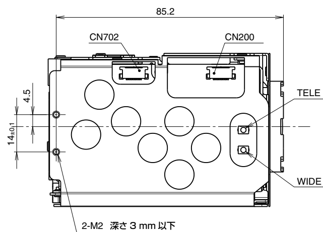
背面
