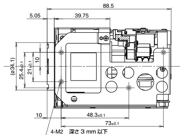
右側面
