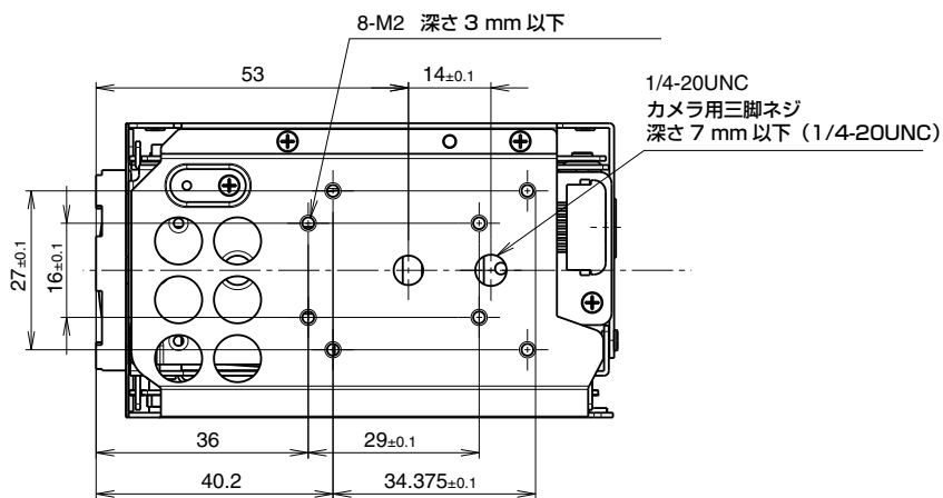
背面
