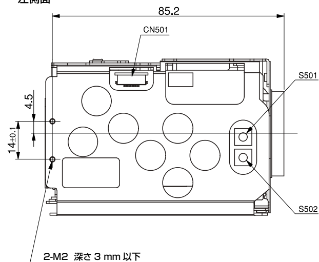
左側面
