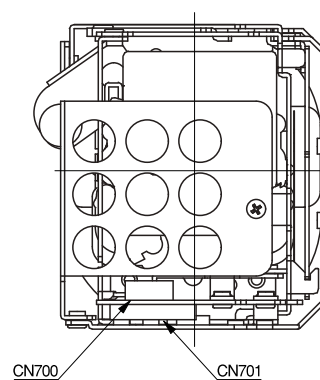
背面
