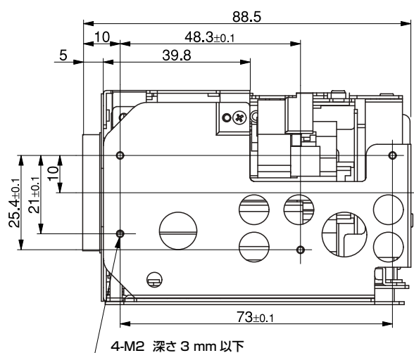
左側面
