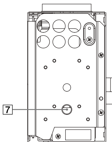
底面
