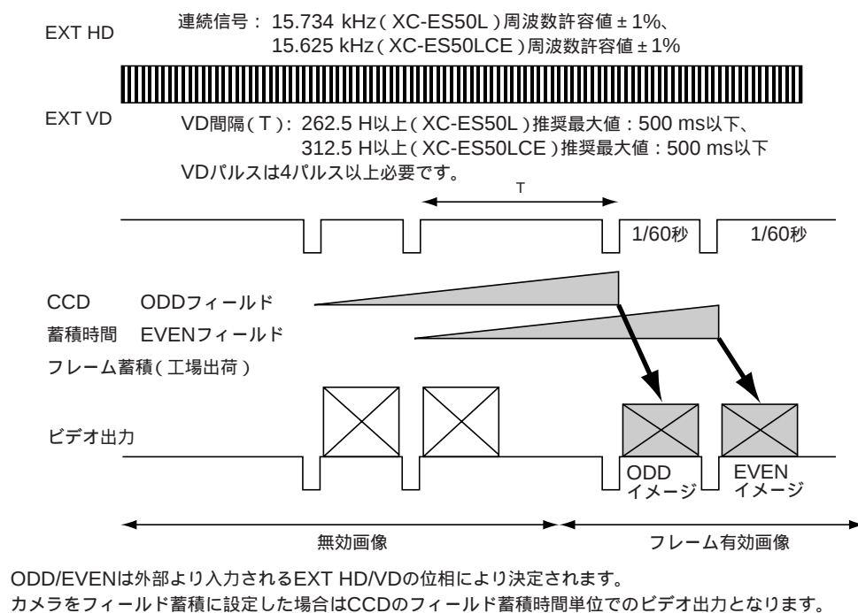
入力タイミングチャート例2
