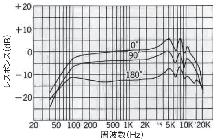
標準周波数特性図
