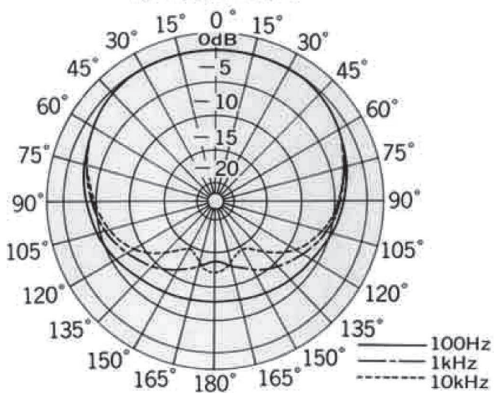
標準指向特性図
