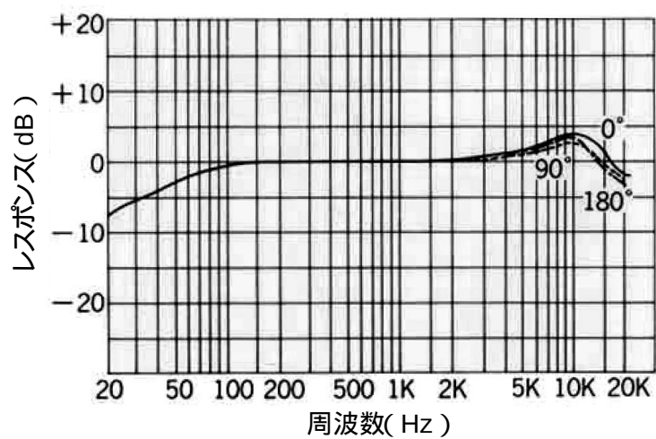
標準周波数特性図
