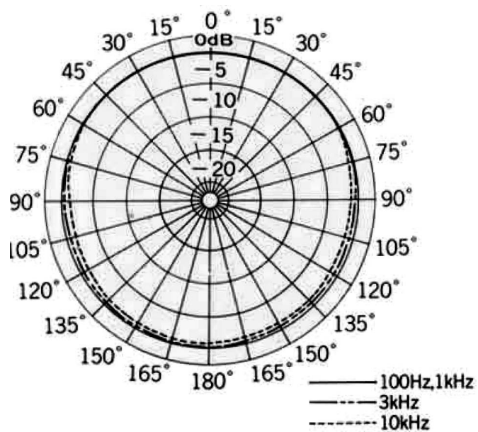
標準指向特性図
