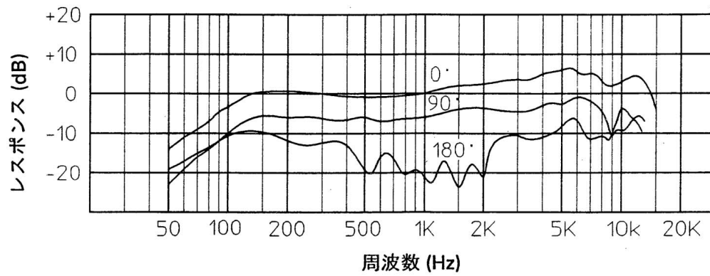
周波数特性
