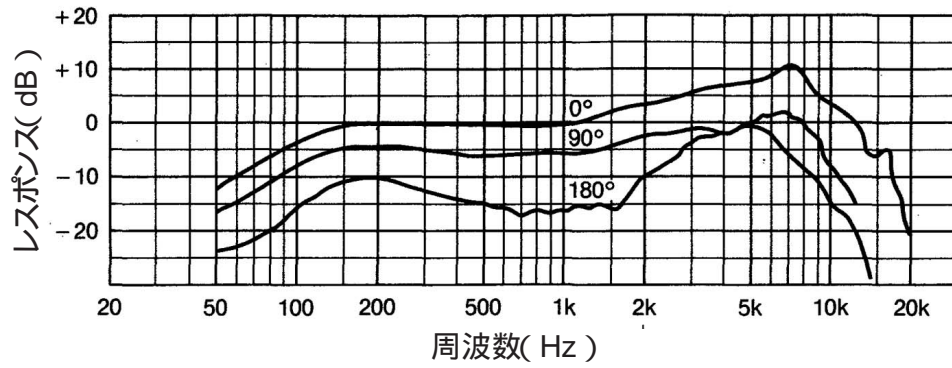
周波数特性
