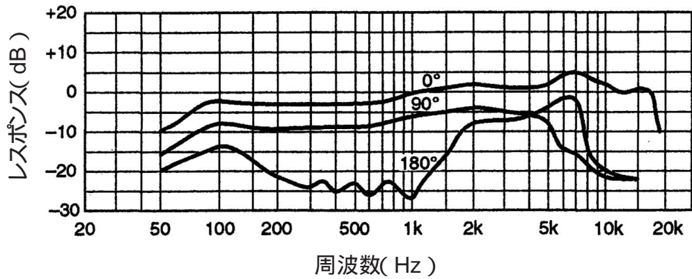
周波数特性
