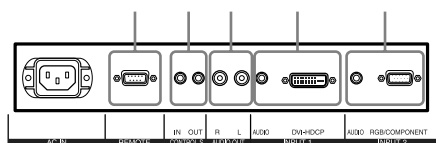
〔底面端子部〕
