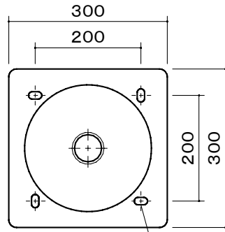
〈A矢視図〉 4-14×25(長穴)
