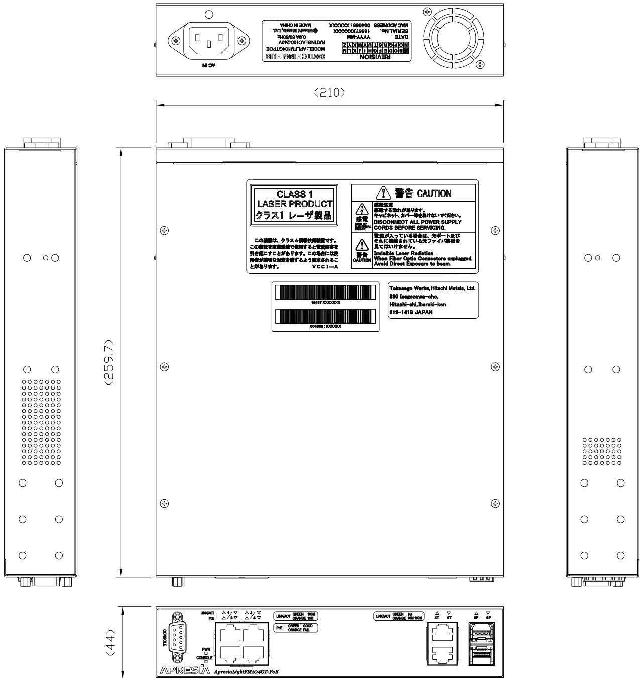
図 11-1 AprasiaLightFM104GT-PoE 外観図
