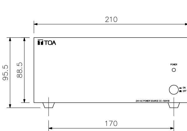
正面図
