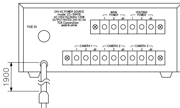
背面図
