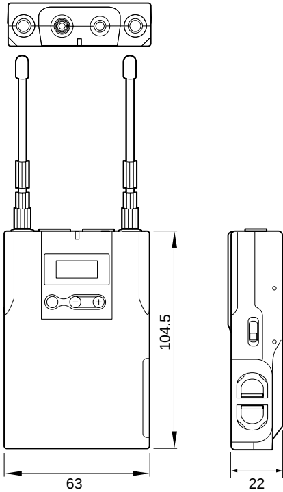
ポータブルダイバーシティチューナー( 受信機 )
