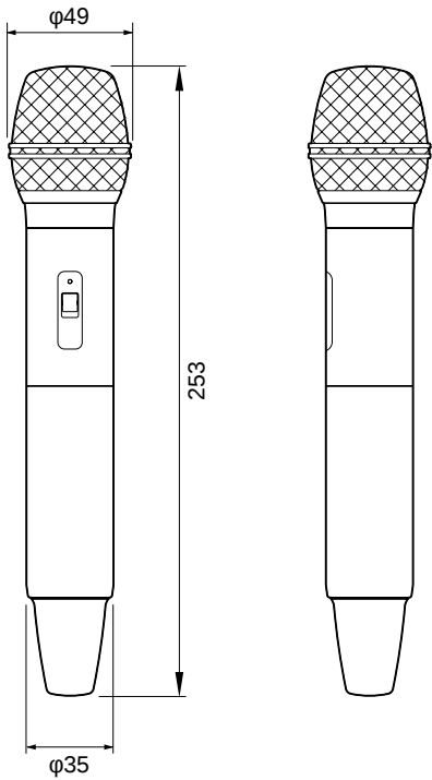
ハンドヘルドトランスミッター( 送信機 )
