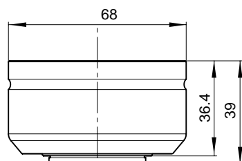
レンズ寸法図
