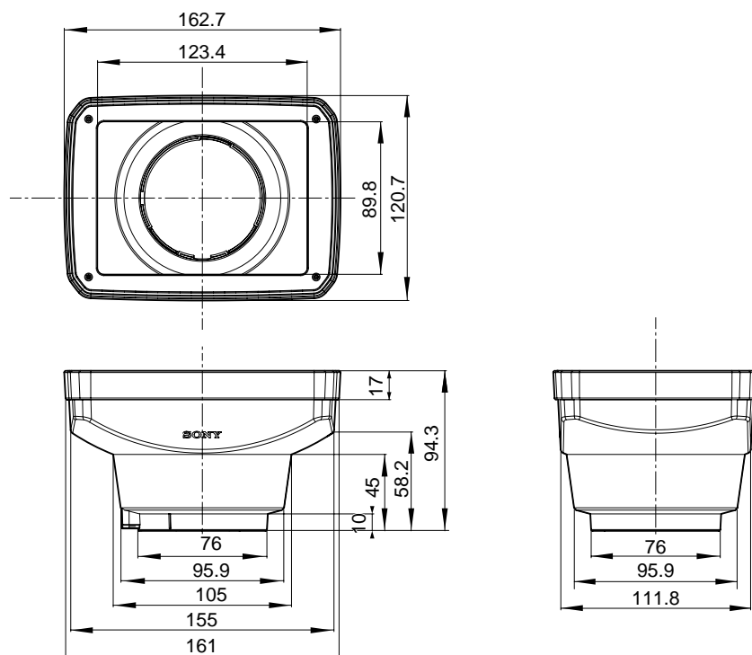
フード寸法図
