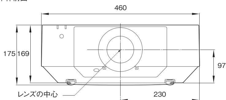
本体前面
