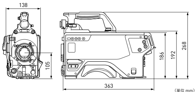
HDC-3500 外形寸法図
