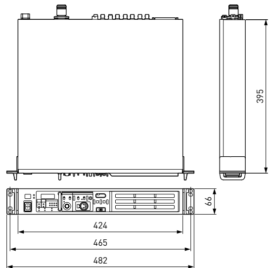
HDCU-3100 外形寸法図
