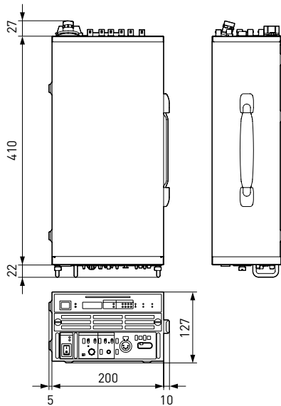
HDCU-3500 外形寸法図
