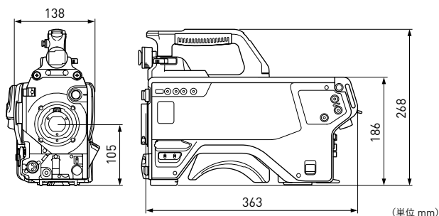
HDC-3100 外形寸法図
