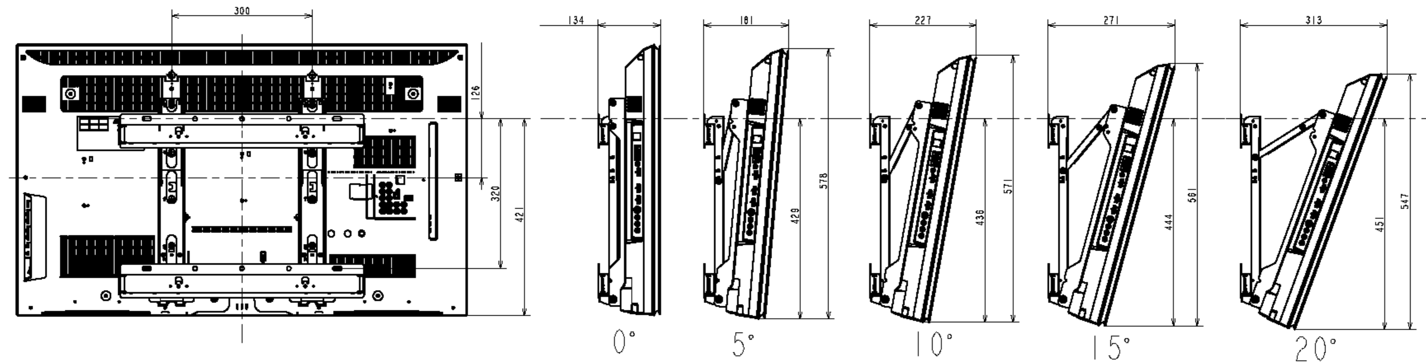
壁掛けユニット 取付け時の寸法図
