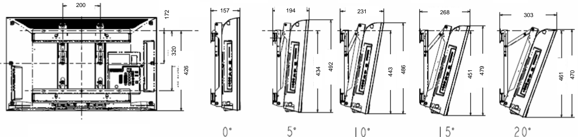
壁掛けユニット 取り付け時の寸法図
