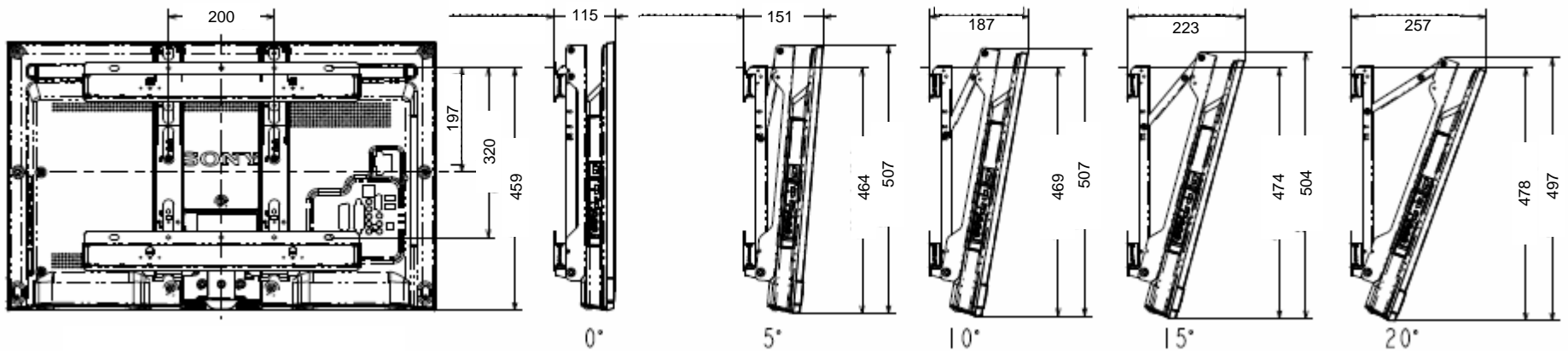
壁掛けユニット 取り付け時の寸法図
