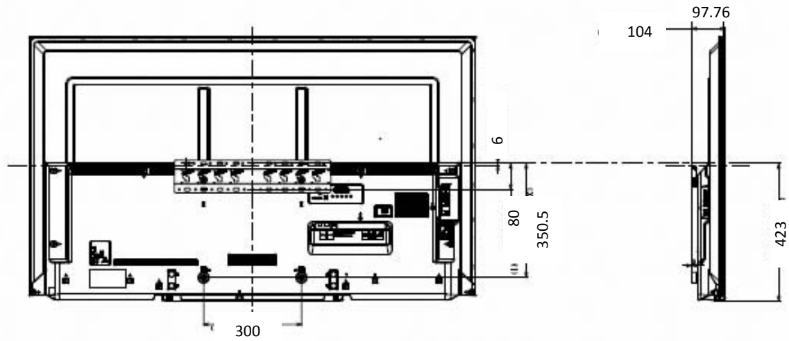
SU-WL450 (SLIM)
