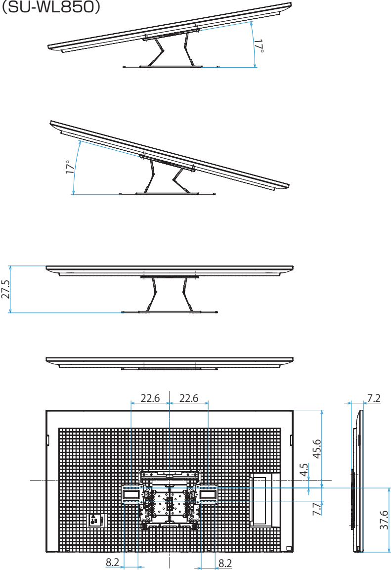
壁掛けブラケット装着時 (SU-WL850)
