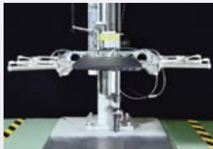
■ 落下試験 落下の衝撃に耐える堅牢性を追求
