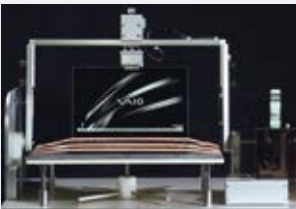
■ 開閉試験 液晶ディスプレイの連続開閉で、数年間の酷使に耐えるヒンジを追求
