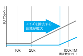
「S-Master HX」のノイズ除去音域(イメージ) ノイズを除去する音域が拡大 10k 20k 100k 1M 周波数(Hz) → — 従来のS-Masterのノイズ分布 — S-Master HXのノイズ分布
